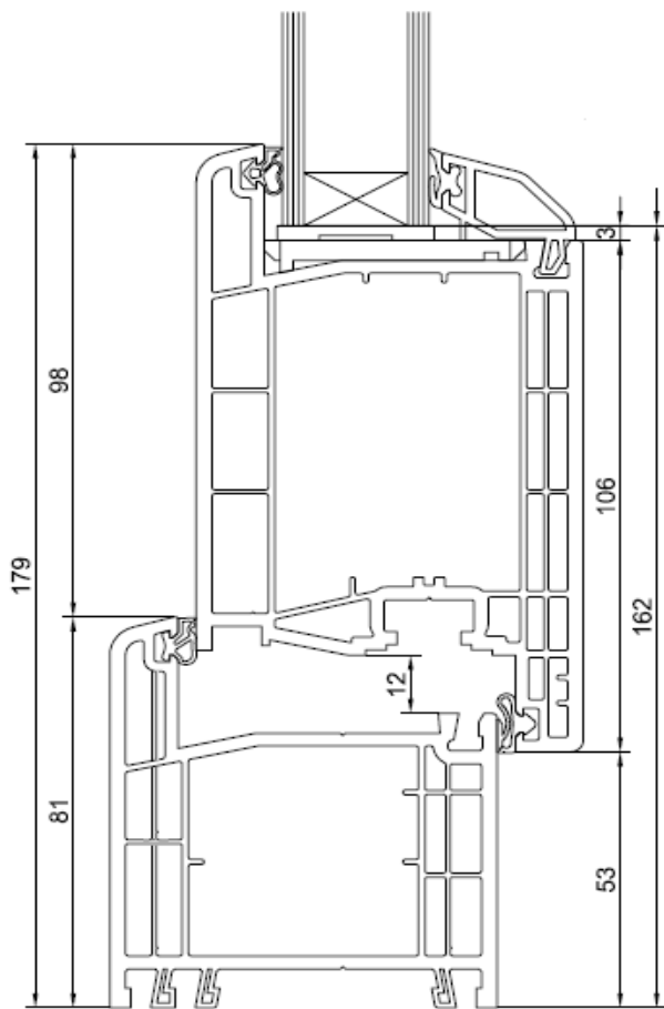
Portoncino Synergic Apertura interna
