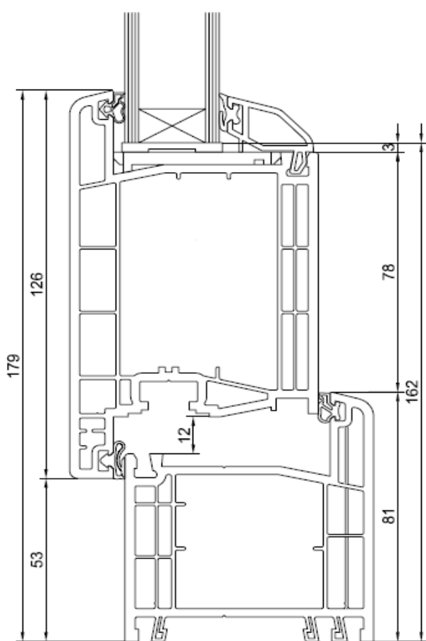
Portoncino Synergic Apertura esterna
